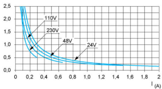
Curvas CA14
