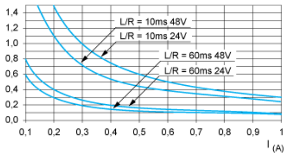
Curvas CC13
