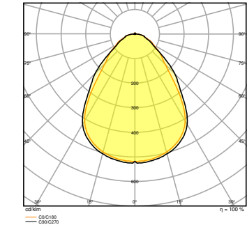
PL CMFT 600 P 33W 865 U19 PS EM CONVERSION BOX
