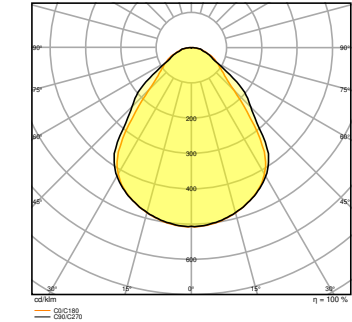
PL CMFT 600 P 28W 865 U19 PS
