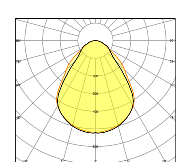
PL CMFT 600 P 33W 865 U19 PS
