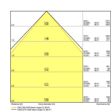
PL CMFT 600 P 28W 865 U19 PS
