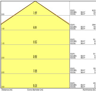
PL CMFT 600 P 33W 830 DALIVR EM
