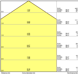
PL CMFT 600 P 33W 830 DALIVR EM CONVERSION BOX
