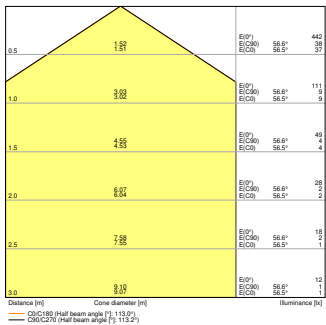
PL CMFT 600 P 33W 865 PS EM
