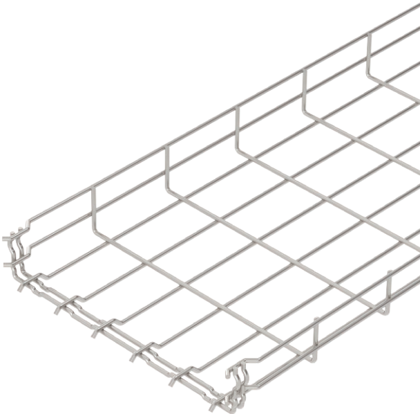
Caminho de cabos em varão com união de encaixe rápido com 55 mm de altura lateral.
