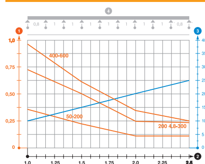
Diagrama de cargas do caminho de cabos GR-Magic do tipo GRM 55
