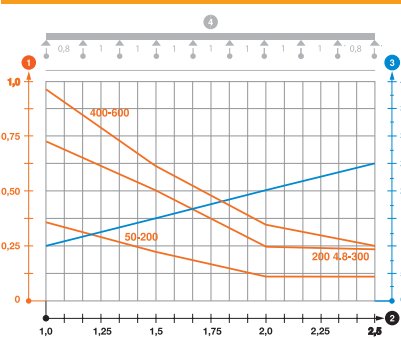
Diagrama de cargas do caminho de cabos GR-Magic do tipo GRM 55
