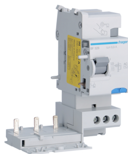
BF326
