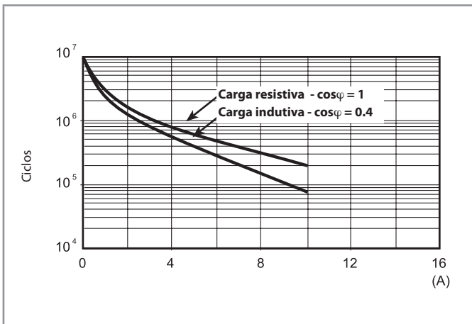
F 40.5 - Vida elétrica (AC) versus corrente nos contatos Tipo 40.11 (página 5)
