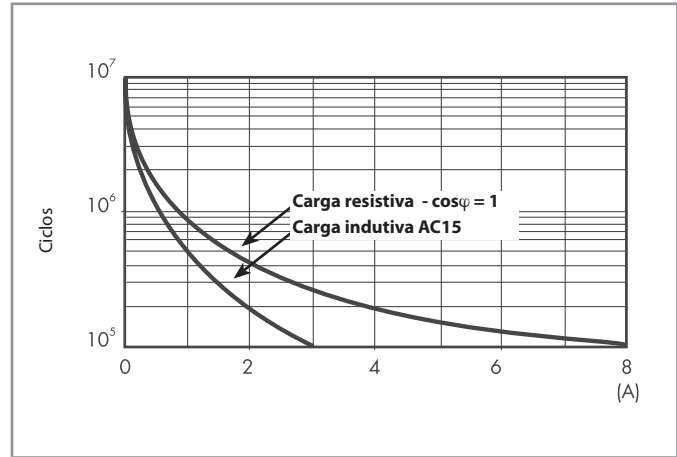
F 40.4 - Vida elétrica (AC) versus corrente nos contatos Tipo 40.52 (página 4)
