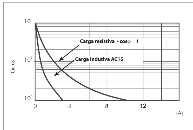
F 40.6 - Vida elétrica (AC) versus corrente nos contatos Tipo 40.62 (página 5)
