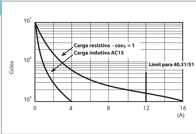
F 40.3 - Vida elétrica (AC) versus corrente nos contatos Tipos 40.31/51/61 (página 4)
