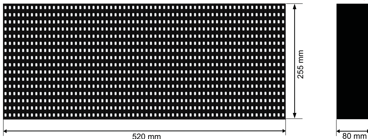
Fig. 3 DISCRSE dimensions
