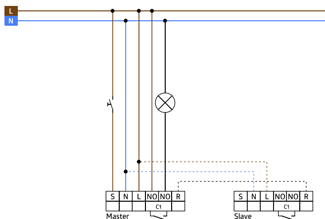
Esquemas elétricos
