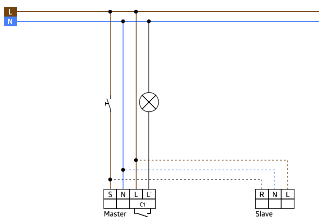
Wiring diagrams
