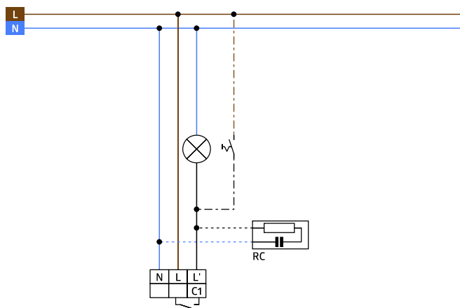
Wiring diagramms
